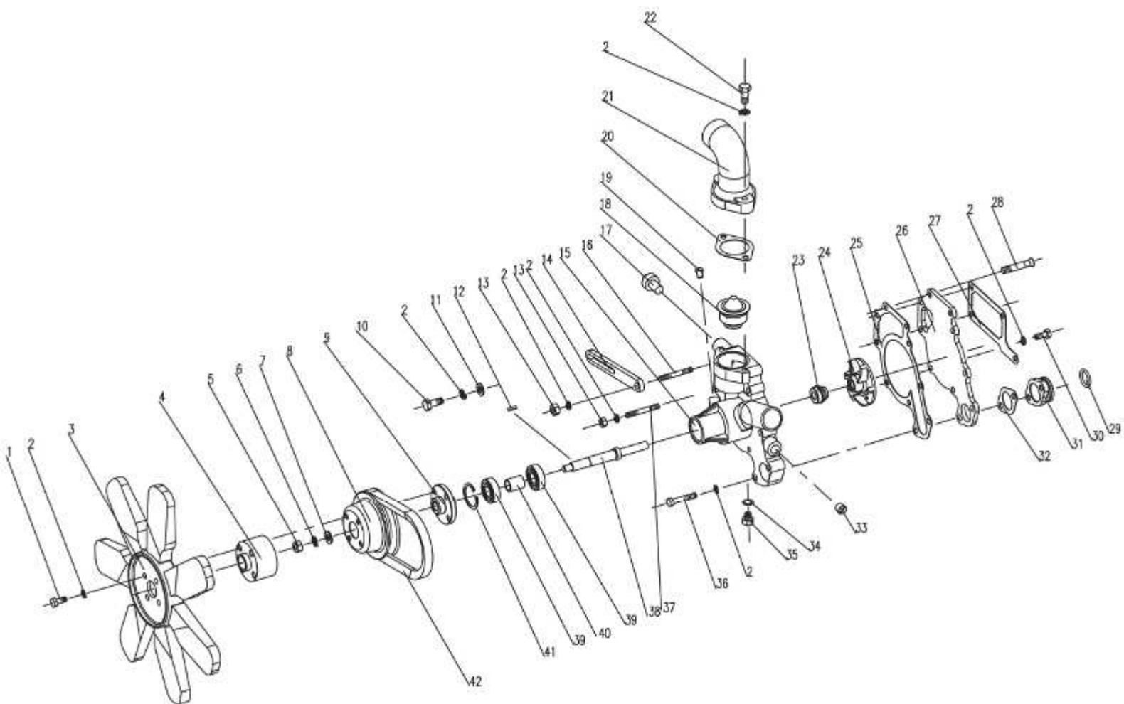
图8 水泵风扇总成
