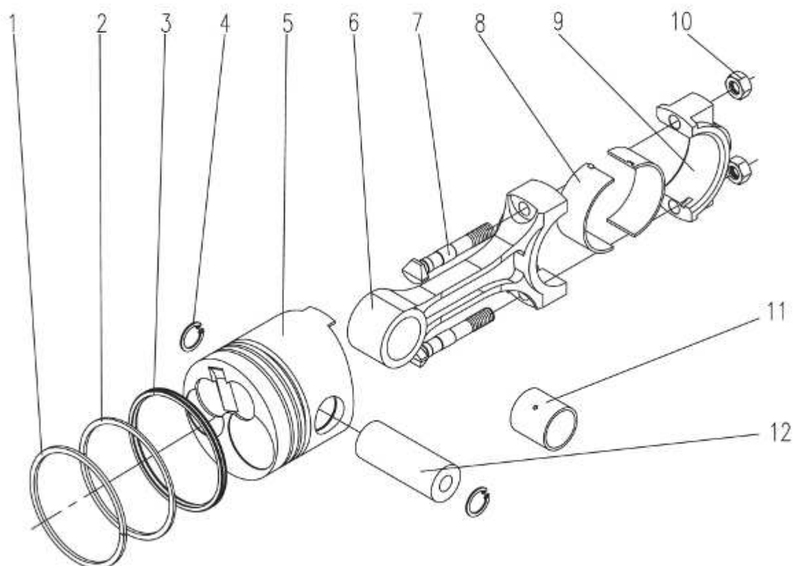
图5 活塞、连杆总成
