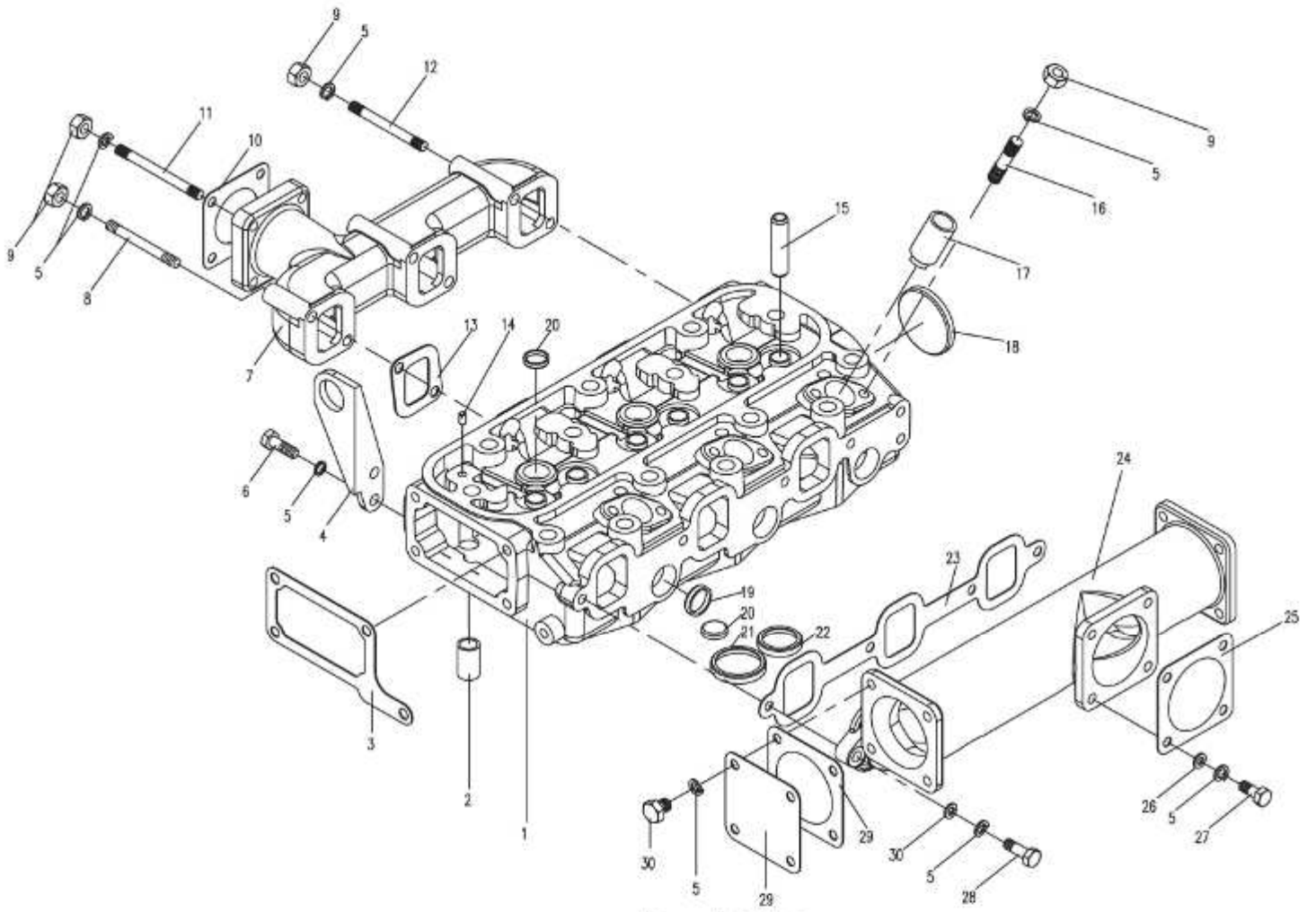
图2 气缸盖总成
