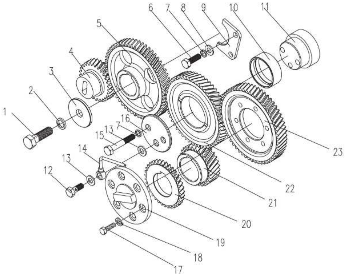
图4 正时齿轮系总成 Fig.4 Timing gear train
