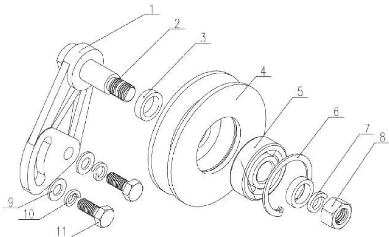
图15 张紧轮部件
