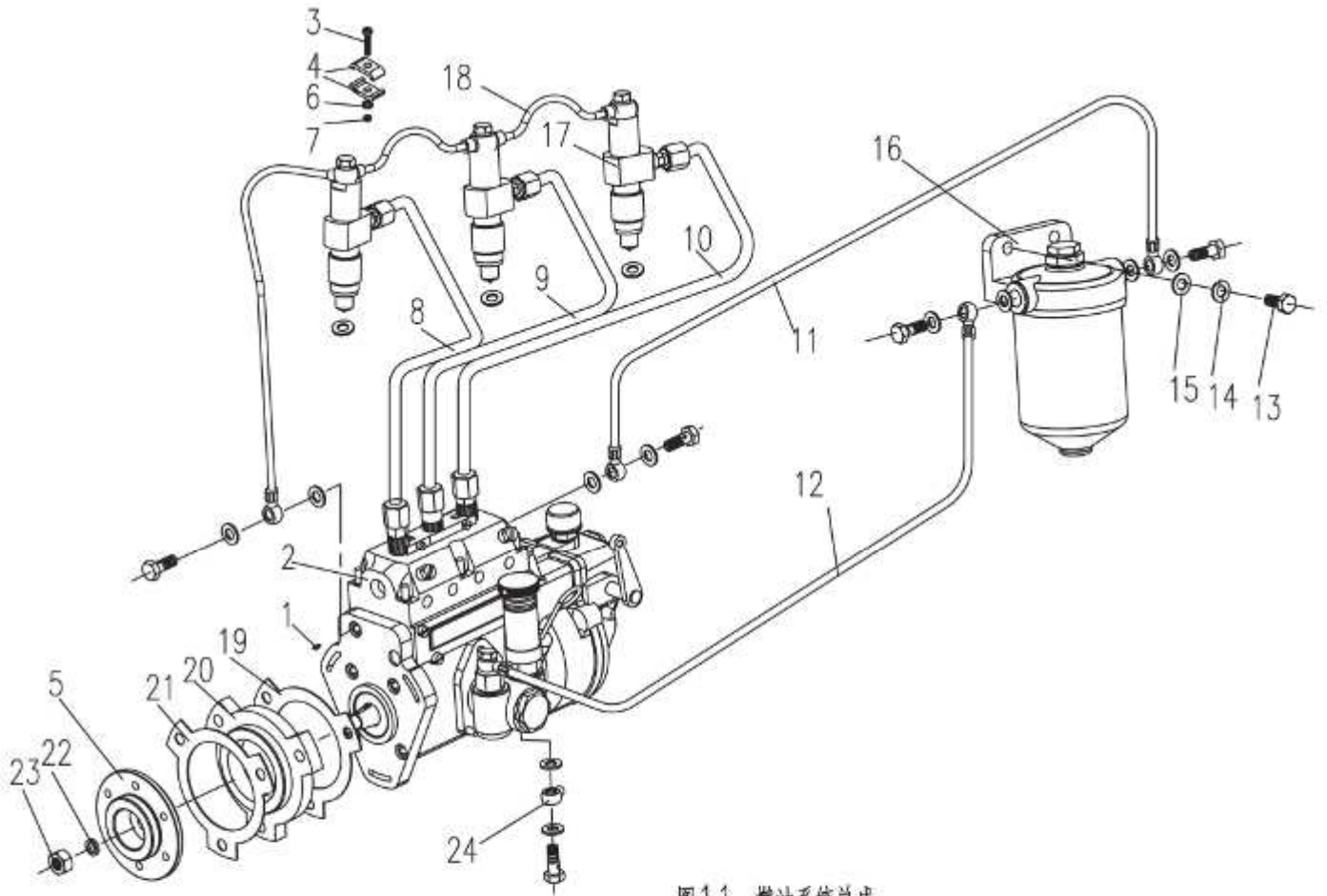
图11 燃油系统总成
