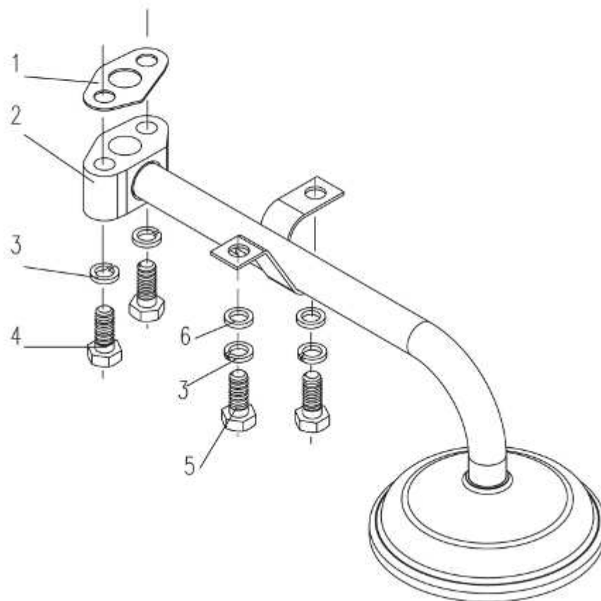
图12 机油集滤器总成
