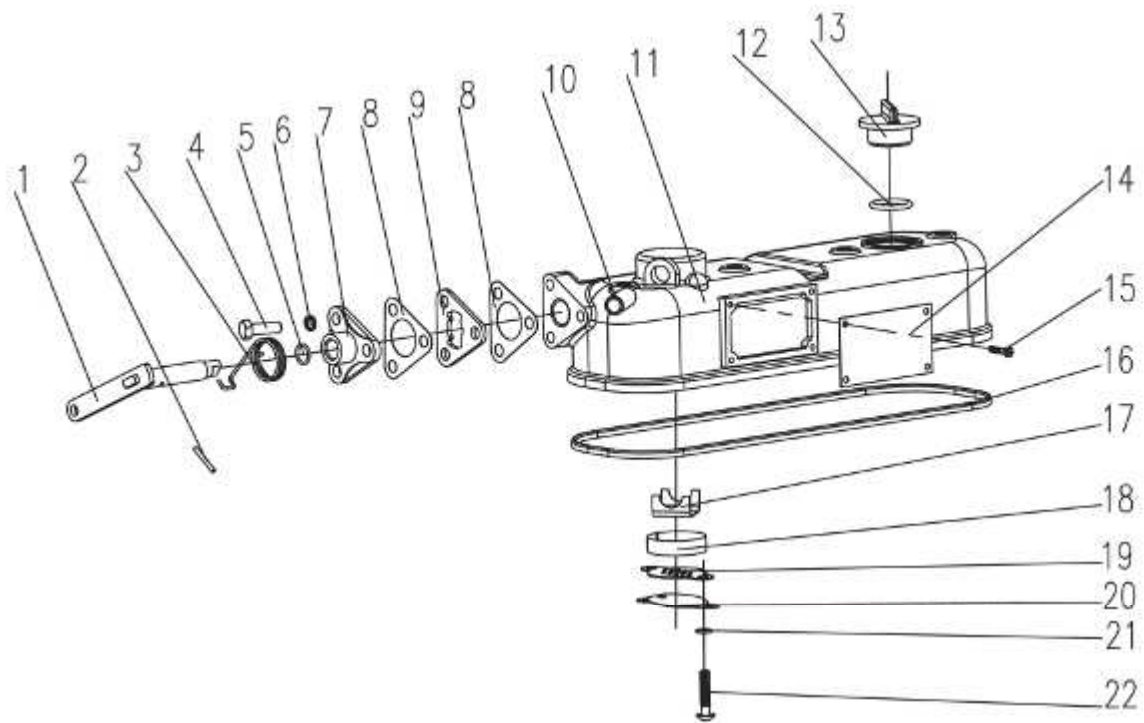
图1 气缸盖罩总成
